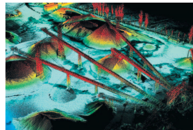
Impianto Conglomerati Bituminosi: restituzione nuvola di punti per calcolo volumetrie dei cumuli
